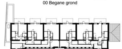
01 eerste verdieping
